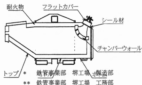
図1 GFコンバータ炉体 Fig.1 GF Converter vessel
