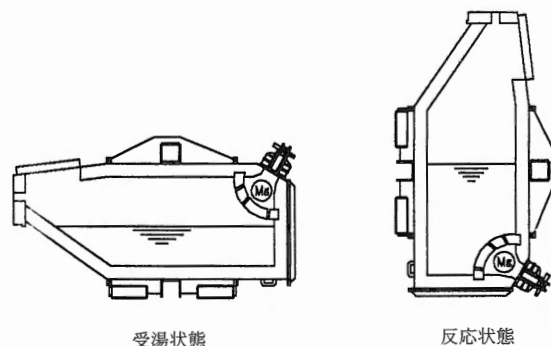
図2 GFコンバータ処理方法 Fig.2 Spheroidal treatment in GF converter
