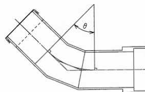
図2 角度( 30^\circ < \theta \leq 60^\circ )の同質曲管
