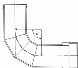
図1 角度( 60^\circ < \theta \leq 90^\circ )の同質曲管
