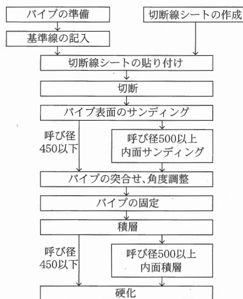
図11 同質曲管の製造フロー
