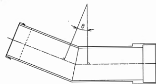
図3 角度( 0^\circ < \theta \leq 30^\circ )の同質曲管
