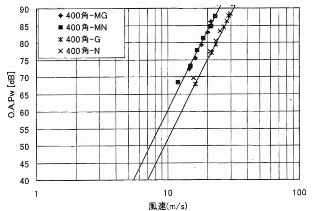
図15 試験結果 送風ガイドの比較
