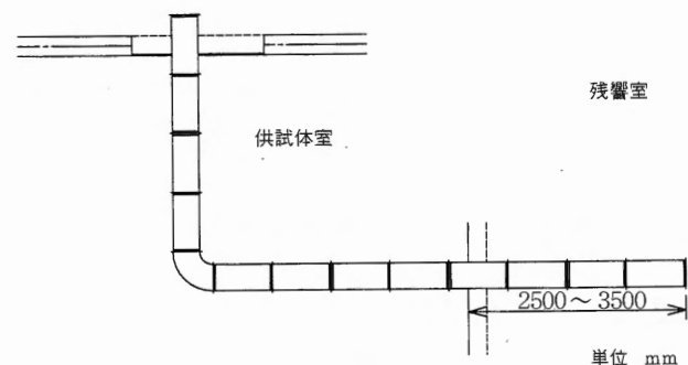
図8 試験装置 ダクト系（B）
