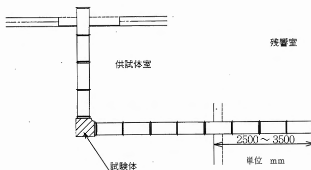
図7 試験装置 ダクト系（A）
