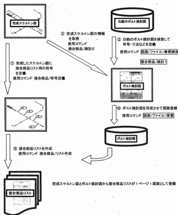
図17 接合部リスト・ボルト検討図の作成
