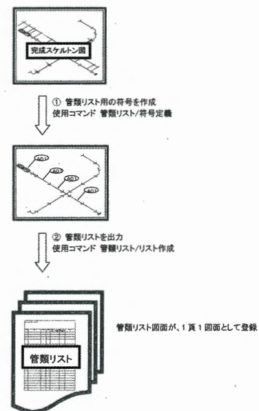
図16 管類リストの作成
