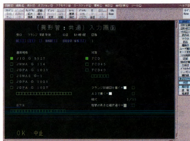
図11 異形管作図入力画面（共通）
