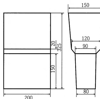
図1 t80テストブロックの形状
