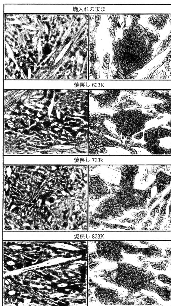
図7 20%Cr-3.43%C（過共晶）における光学顕微鏡組織 Fig. 7 Optical micrographs of 20%Cr-3.43%C(hypereutectic)
