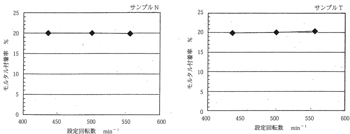
図9 モルタル付着率 Fig. 9 Adhesion rate of mortar
