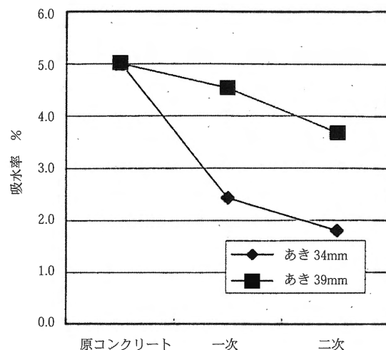
図5 吸水率
