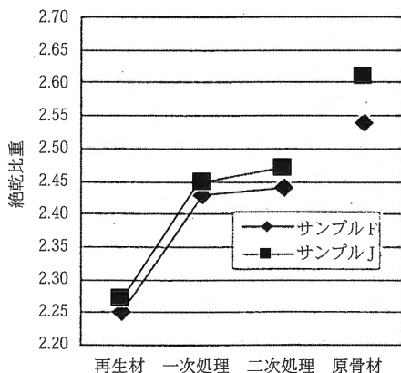
図10 絶乾比重
