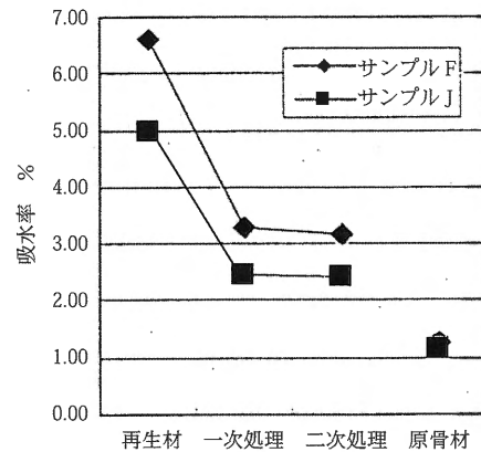
図11 吸水率
