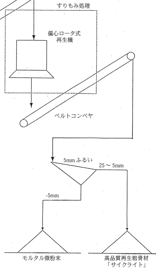
図1 実験設備のフロー
