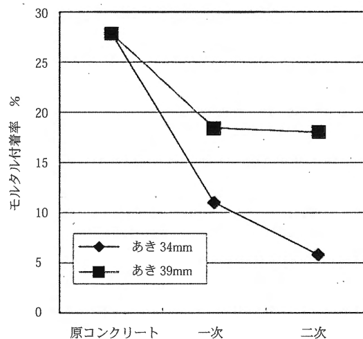
図6 モルタル付着率
