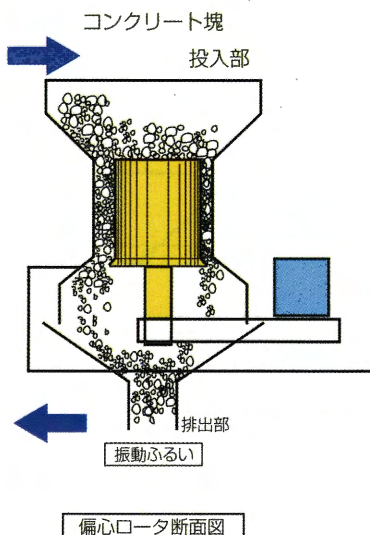
図3 再生機の断面図
