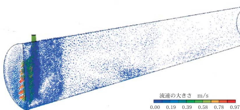
図6 速度ベクトル図(集中Ⅱ型模型) Fig. 6 Velocity vector(combination model II)
