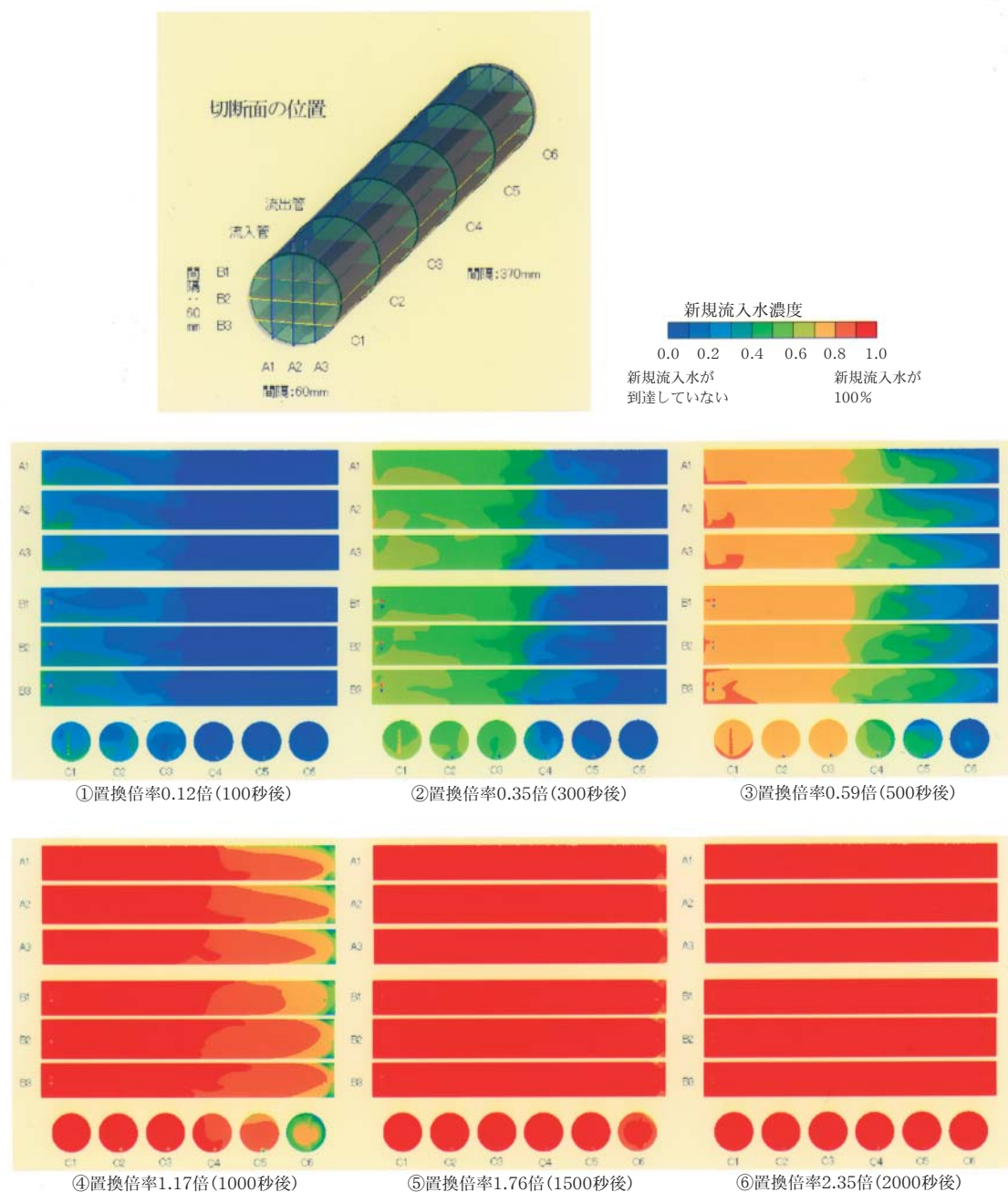
図11 模型貯水槽内の水の入替わり状況(集中Ⅱ型模型) Fig. 11 Simulation of water displacement (combination model II)
