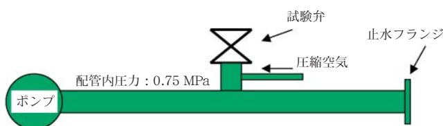
図4 圧力下排気試験装置
