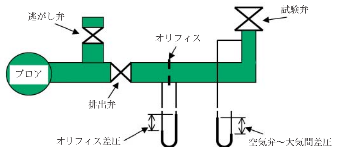
図5 排気量測定試験装置
