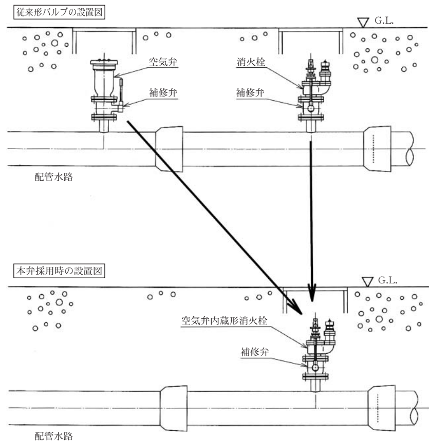
図1 空気弁内蔵形地下式消火栓の設置例
