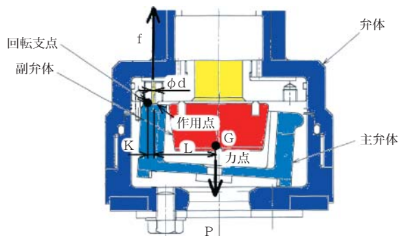
図9 圧力下排気の状態
