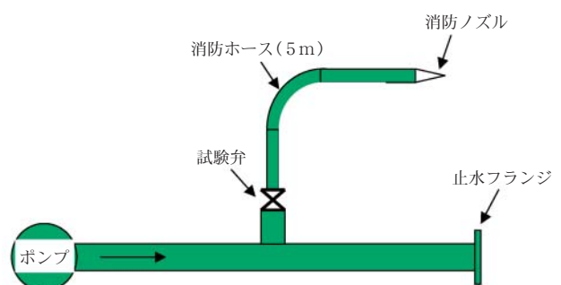
図6 放水量測定試験装置
