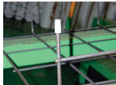
図14. 樹脂製キャップ拡大図 Fig. 14 Resinous cap
