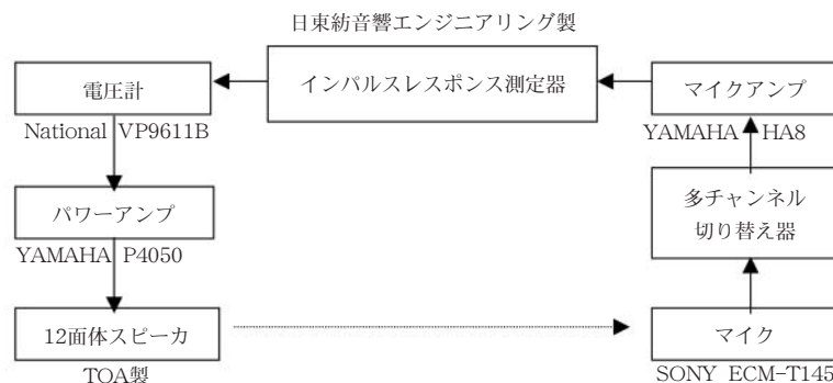
図5 計測装置
