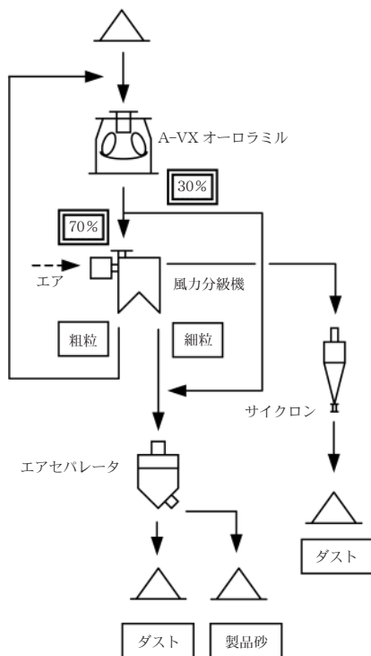
図1 乾式砕砂システムフローシート
