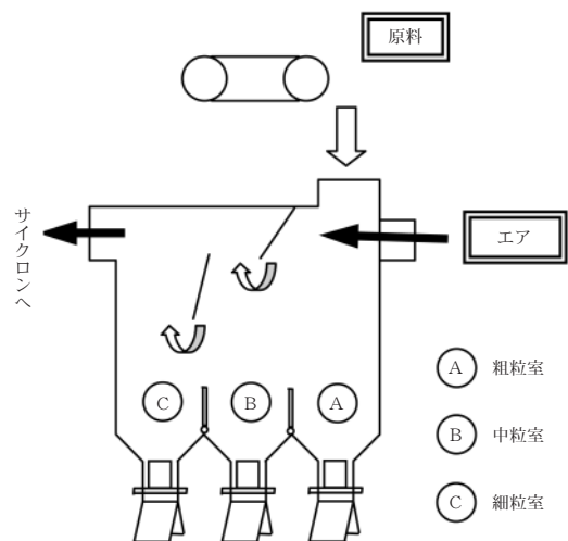
図4 風力分級機模式図 Fig. 4 Schema of air classifier
