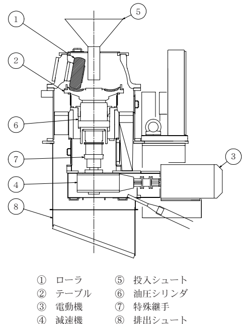
図3 オーロラミルの構造図
