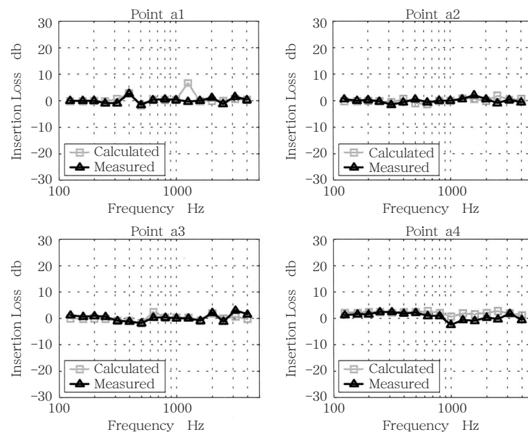
図5 a列における低層遮音壁の実験と計算による挿入損失
