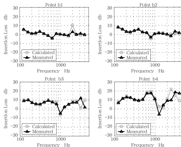
図6 b列における低層遮音壁の実験と計算による挿入損失
