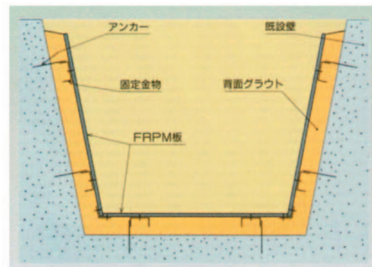
〔施工断面図〕
