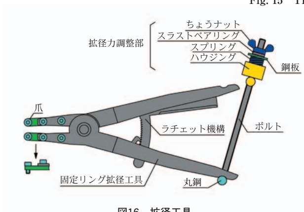
図16 拡張工具 Fig. 16 Expansion tool
