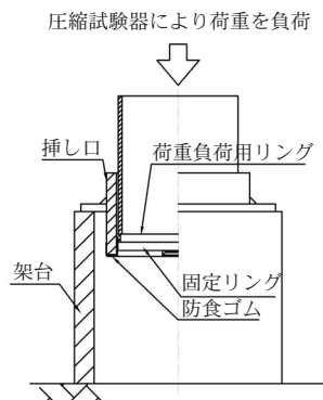
図6 押し抜き抵抗確認試験
