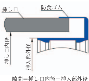
図7 防食ゴムと挿し口との隙間
