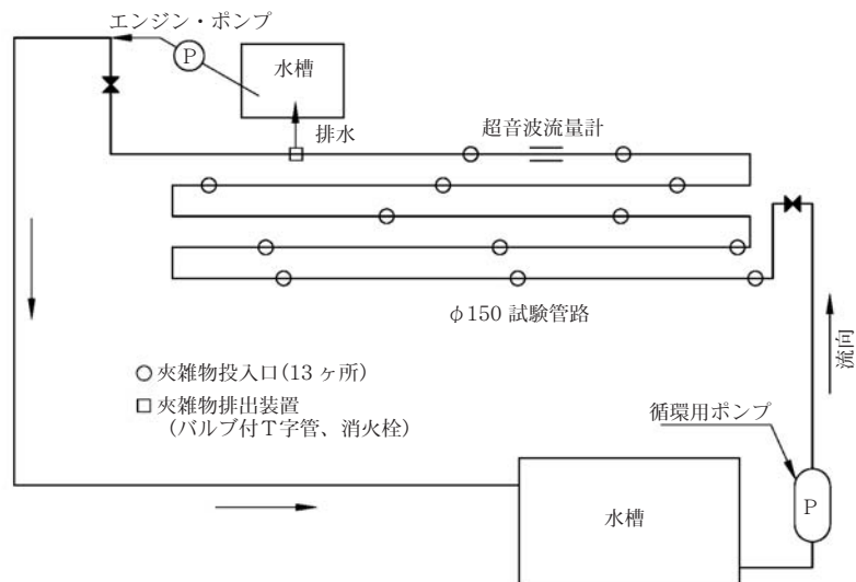
図9 効率的利用方法研究のための実験管路
