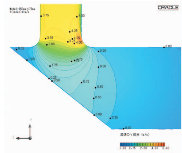
図8 鉛直方向速度分布
