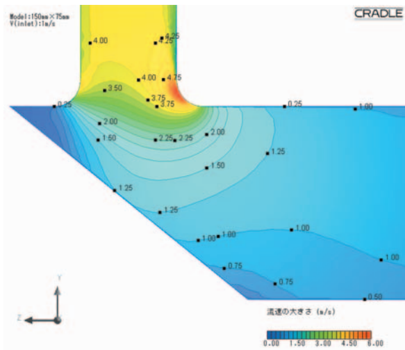
図7 管内流速分布
