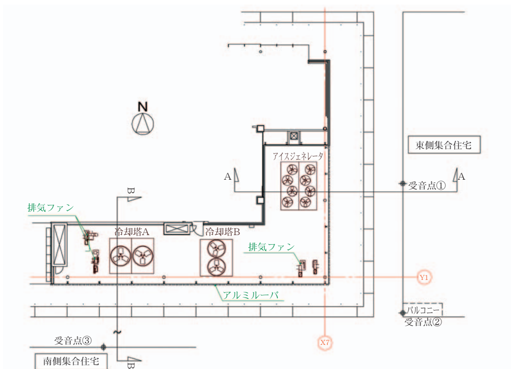
図1 建物概要(7階平面図)
