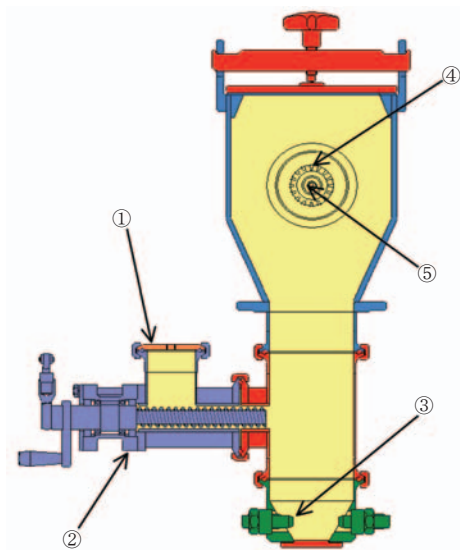
①原料投入口 ②スクリーフフィーダ ③粉碎ノズル ④分級ロータ ⑤粉碎品排出口
