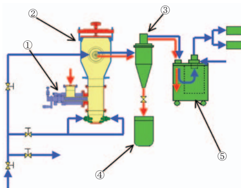
①スクリュフィーダ ②ジェットミル ③サイクロン ④粉砕品回収容器 ⑤バグフィルタ（エジェクタ付き）
