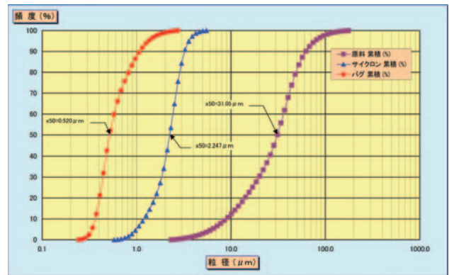
図4 原料および粉碎品の粒度曲線
