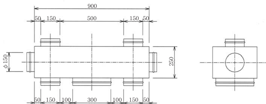
図4 横型楽ボックス Fig. 4 Horizontal "Raku-Box"
