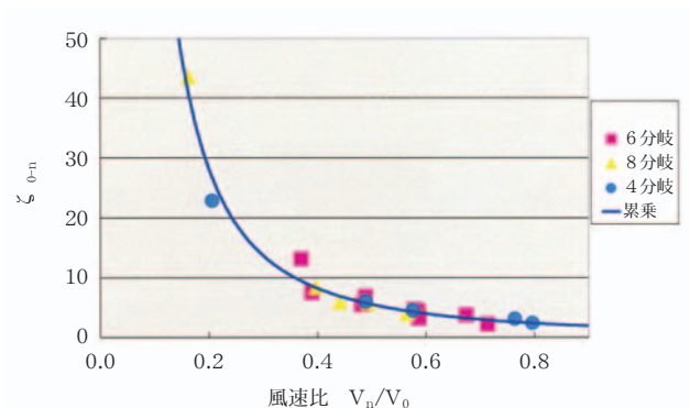
図8 風速比と形状抵抗係数の関係
