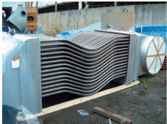
図4 熱交換ユニット Fig. 4 Heat exchanging unit
