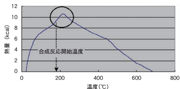
図6 BMA 法による混合体の熱示差分析結果 Fig.6 Result of DTA of mixture by BMA processing
