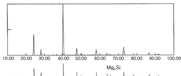
図5 SPS法により得られたバルク体のX線回折結果 Fig.5 X-ray diffraction pattern of bulk compact by SPS processing
