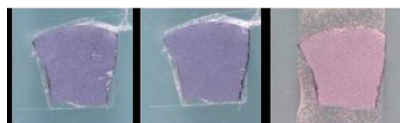
図8 Mg_2Si の塩水噴霧試験結果 (左より試験前、1000h後、2000h後) Fig.8 Results of Mg_2Si salt-spray test
