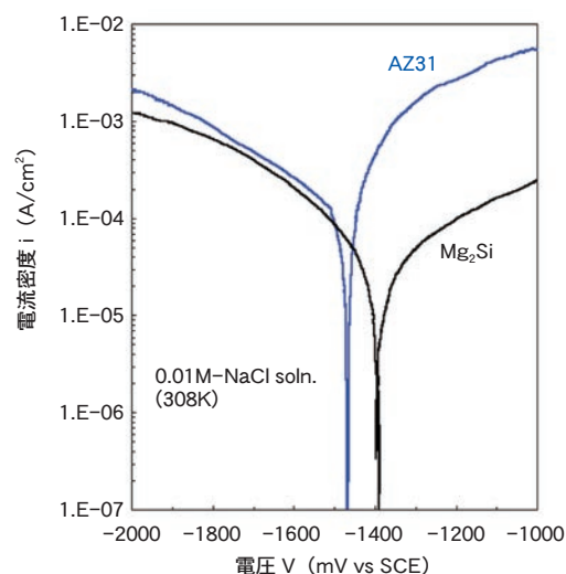
図7 Mg_2Si の分極特性曲線 Fig.7 Polarization curve of Mg_2Si
