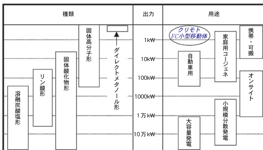
図1 燃料電池の種類と利用分野 1)
