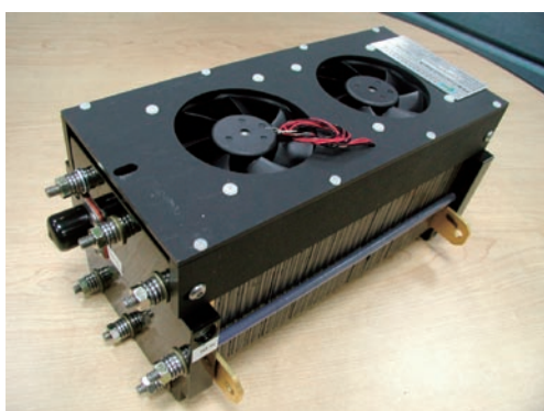
図6 車いす向け空冷式250W燃料電池スタック Fig.6 Air cooling 250W fuel cell stack for wheelchair
