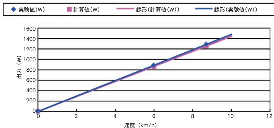
図3 速度と出力の関係
