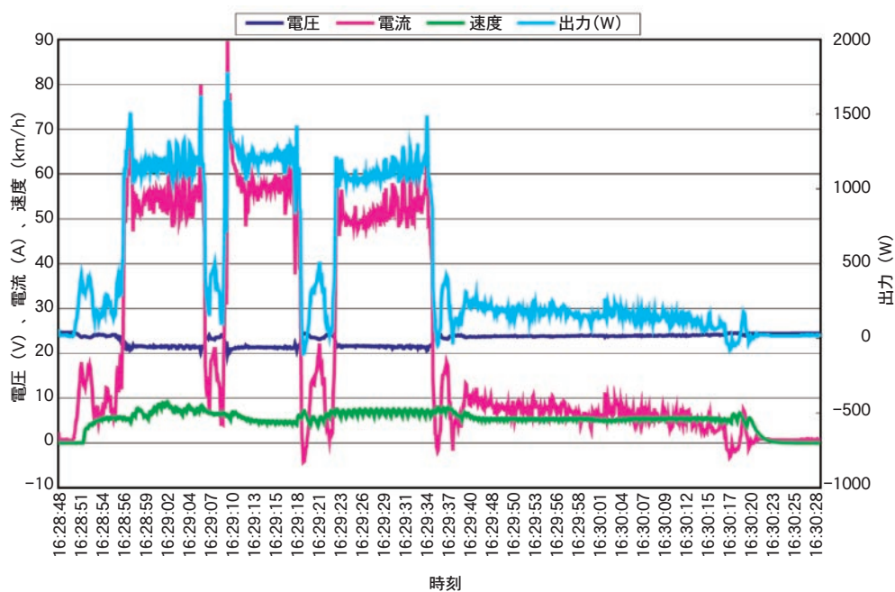
図5 車いすの走行特性、登坂(max)時の電池電圧、電流特性、斜度：約15°
