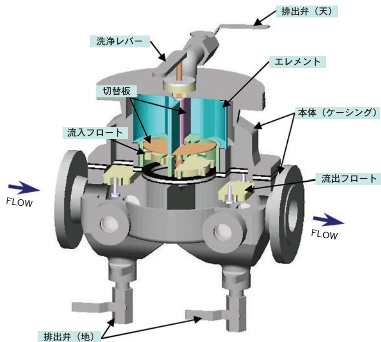
図1 インラインフィルター概略図
