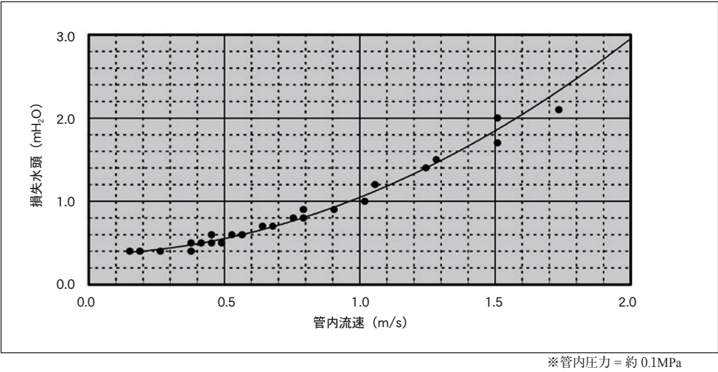
図8 損失水頭実測値と近似曲線
