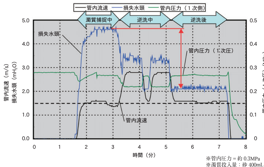
図9 逆洗効果の確認結果(測定チャート)
