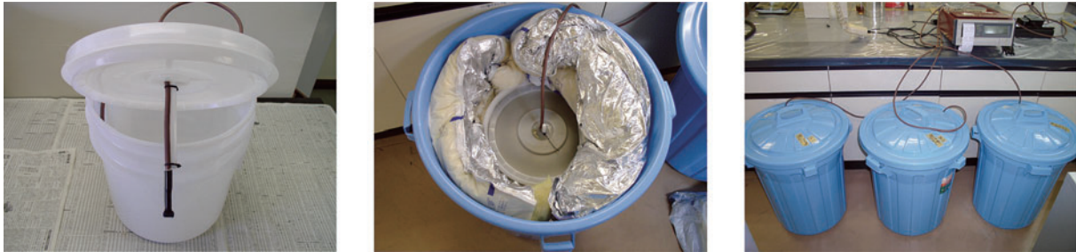
図7 硬化熱測定
