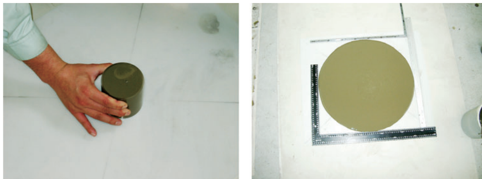
図2 フロー値試験
