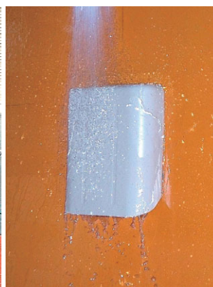
図12 試験風景(2)
