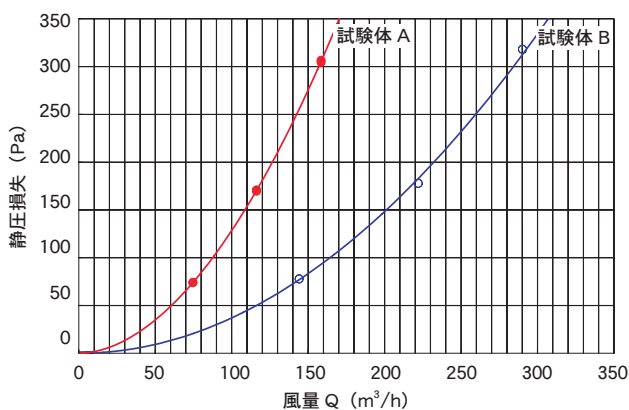
図5 P-Q線図
