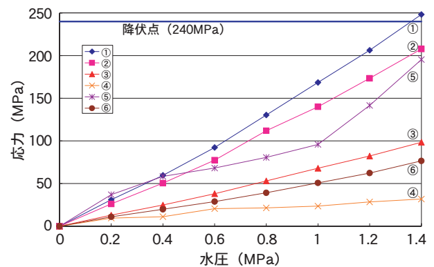
図8 応力測定結果
