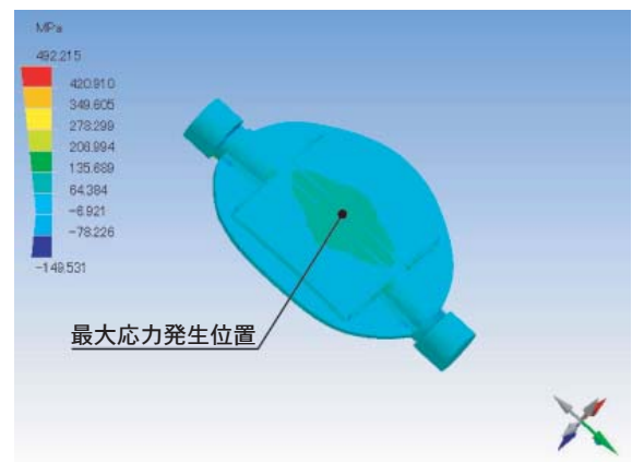
図9 FEM解析結果(呼び径φ750)
