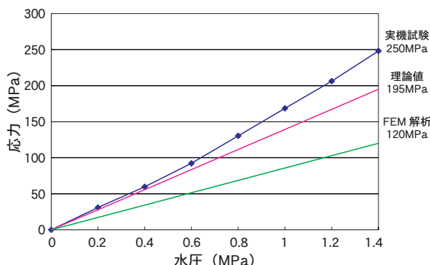
図16 弁体発生応力の比較(呼び径 \phi 750 )
