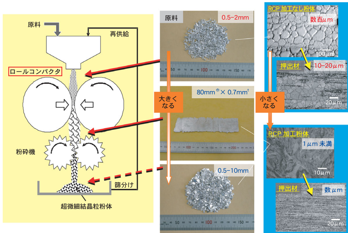
図1 高強靱性Mg合金部材製造技術(RCP工法)の原理
