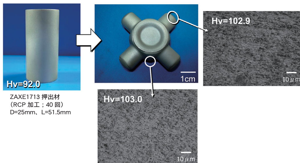
図8 鍛造部材のサンプルおよび組織写真
