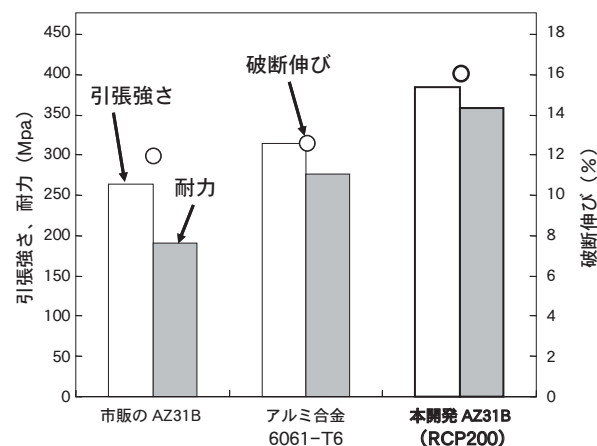
図6 引張特性と破断伸びの比較
