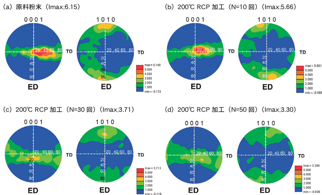
図7 底面配向性のランダム化に関する検討結果
