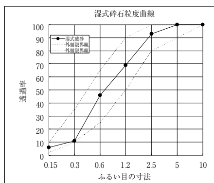
湿式破砂
