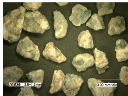
図4 既設湿式砕砂 (2.5~1.2mm)
