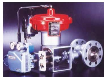
図3 偏心回転プラグ弁
