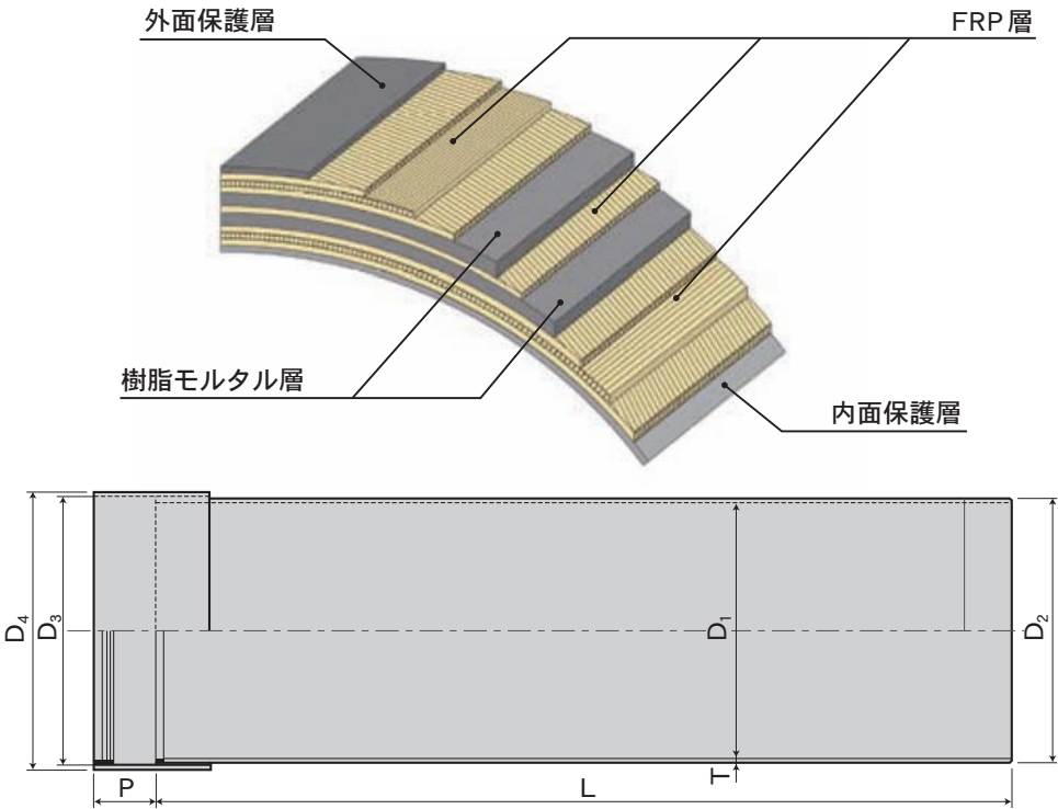
薄肉ポリコンFRP管の形状及び寸法
